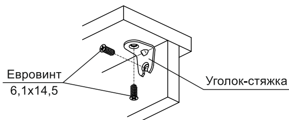
Схема 3. Установка уголка-стяжки
