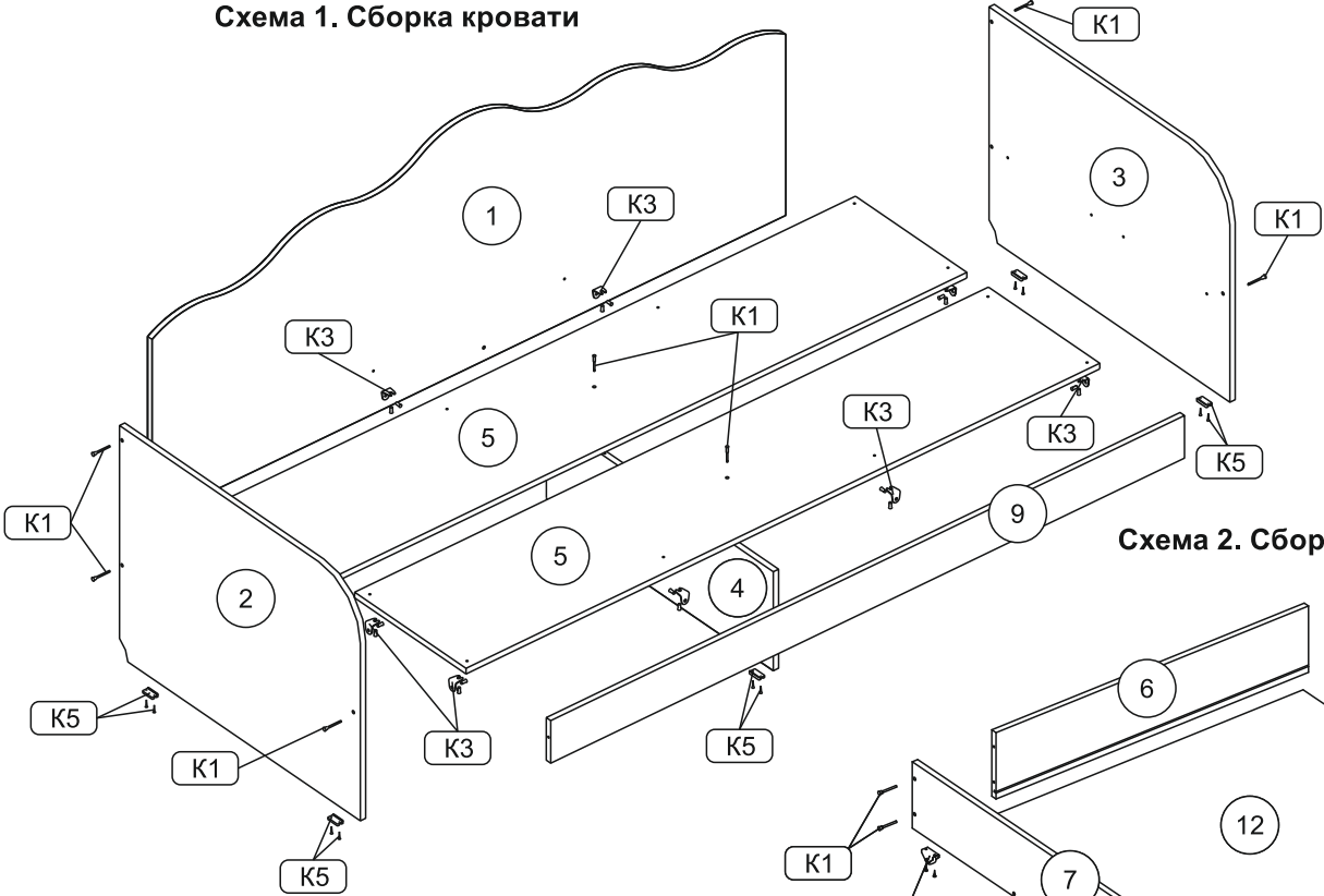
Схема 1. Сборка кровати
