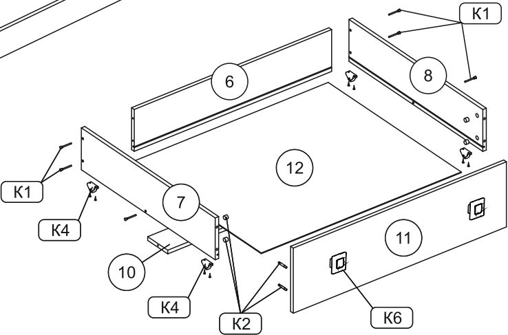
Схема 2. Сборка ящика
