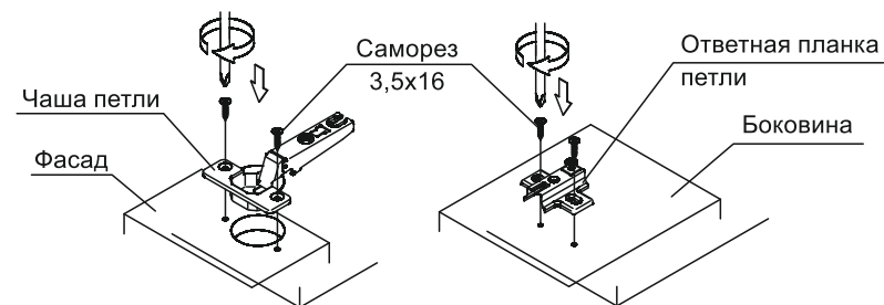
Схема 3. Установка петель
