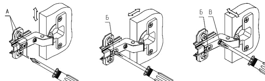
Схема 4. Регулирование положения фасада
