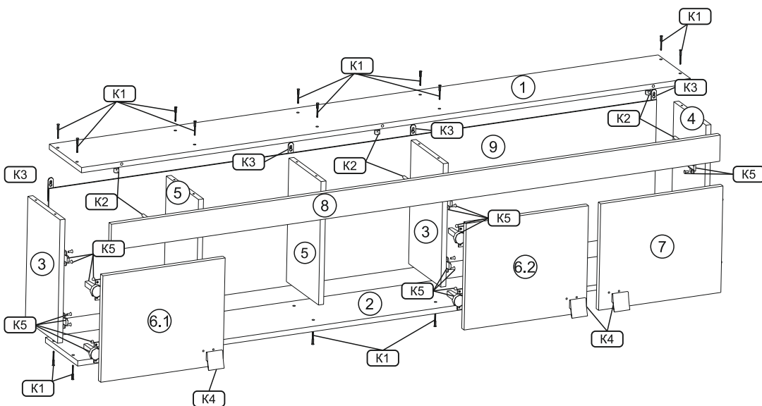
Схема 1. Сборка полки
