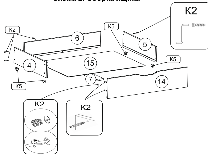
Схема 2. Сборка ящика
