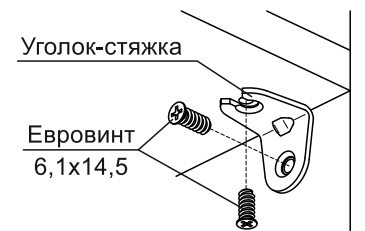
Схема 3. Установка уголка-стяжки
