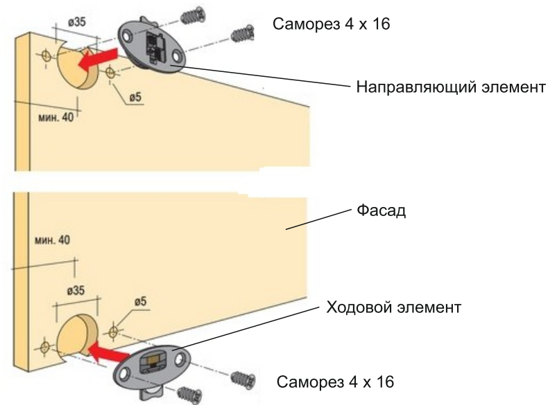
Схема 3. Установка и регулировка ходовых элементов
