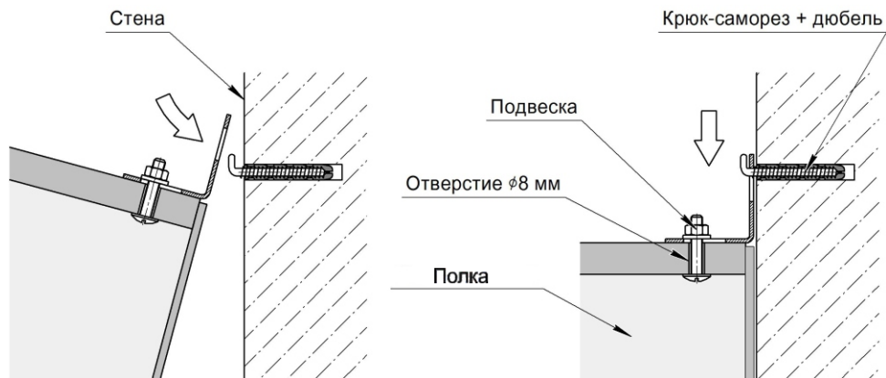
Схема 2. Навеска полки на стену
