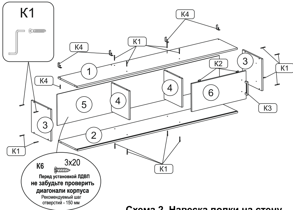
Схема 2. Навеска полки на стену
